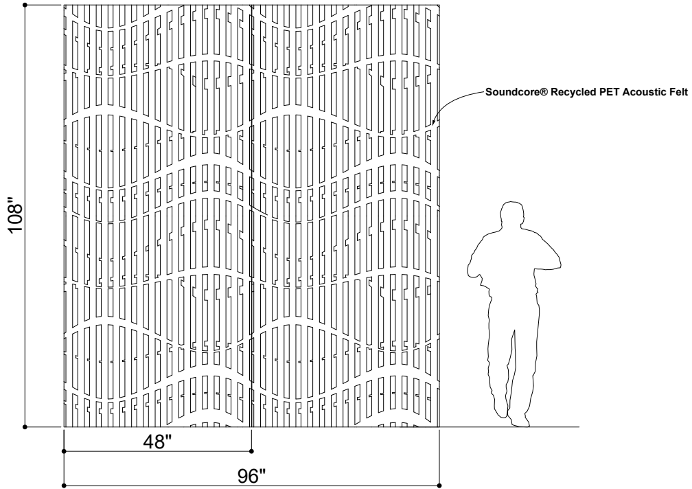
① ELEVATION 1
